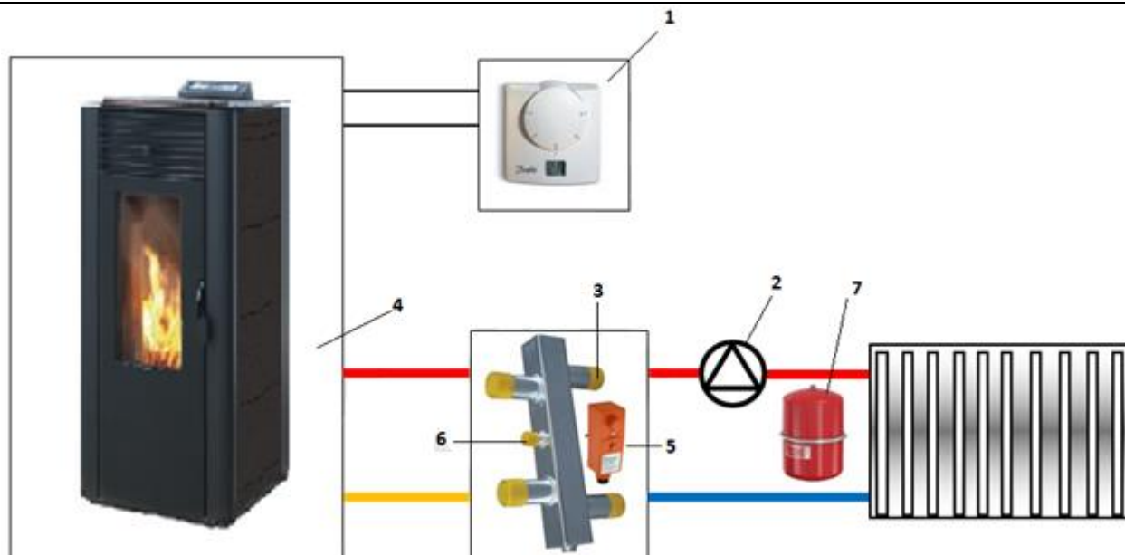
Moederhaard in combinatie met open verdeler (alleen verwarming)
